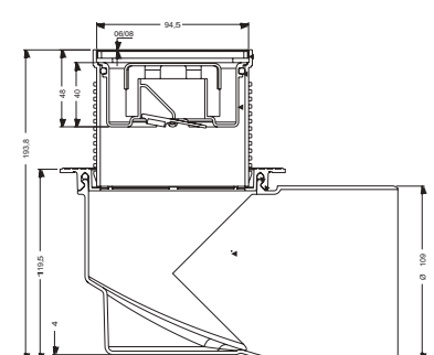
Ø 100 HORIZONTAL OUTLET
