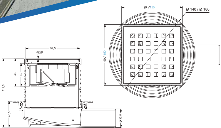
Ø 32 HORIZONTAL OUTLET
