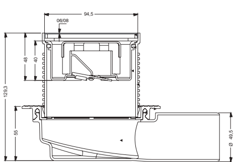
Ø 50 HORIZONTAL OUTLET
